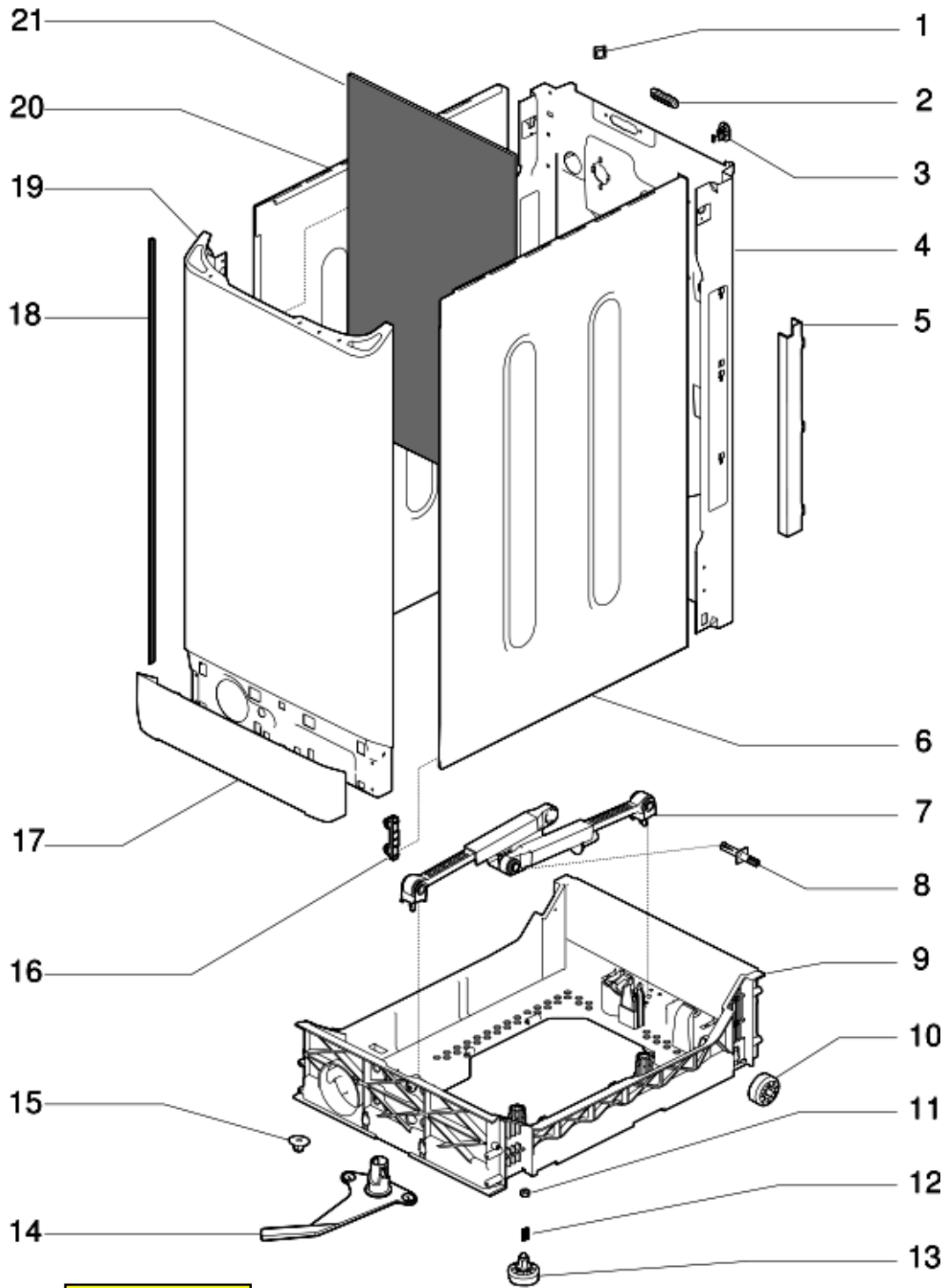
VUE A
