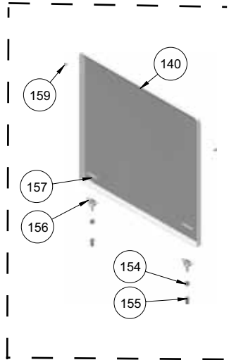
METAL LID OPTIONAL (POSITION NO 153)
