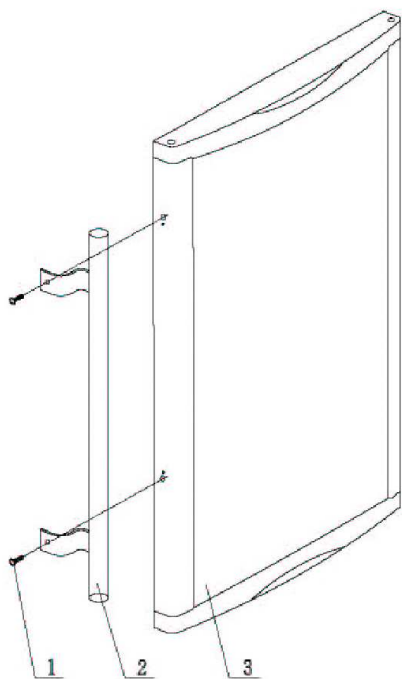
1. Vis 2. Poignée 3. Porte
